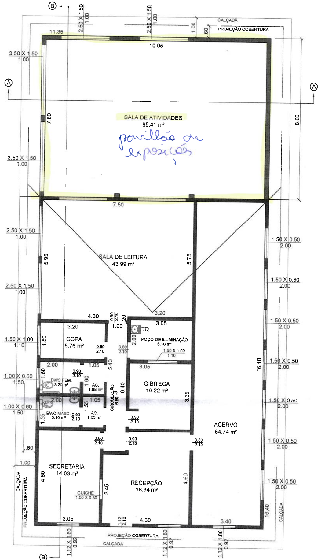
PLANTA BAIXA ESC. 1:100
