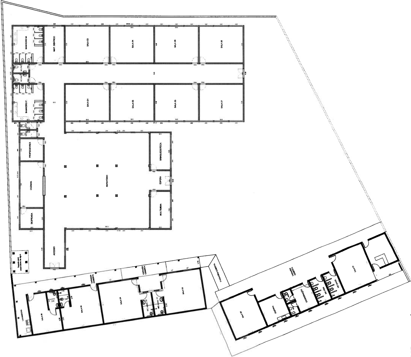
PLANTA BAIXA - SITUAÇÃO PROPOSTA Escala: 1:120
