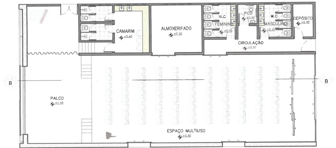
PLANTA ESPAÇO MULTIUSO – PROPOSTA ESC. 1:125
