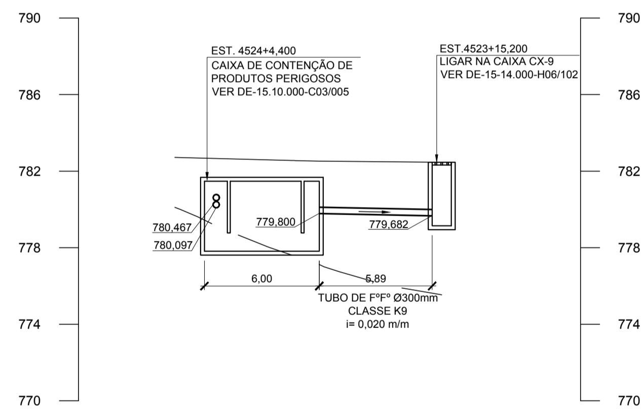
PERFIL DA LIGAÇÃO DA REDE DE DRENAGEM DO TÚNEL 401 COM DRENAGEM DA VIA - ESTACA 4523+15,200
