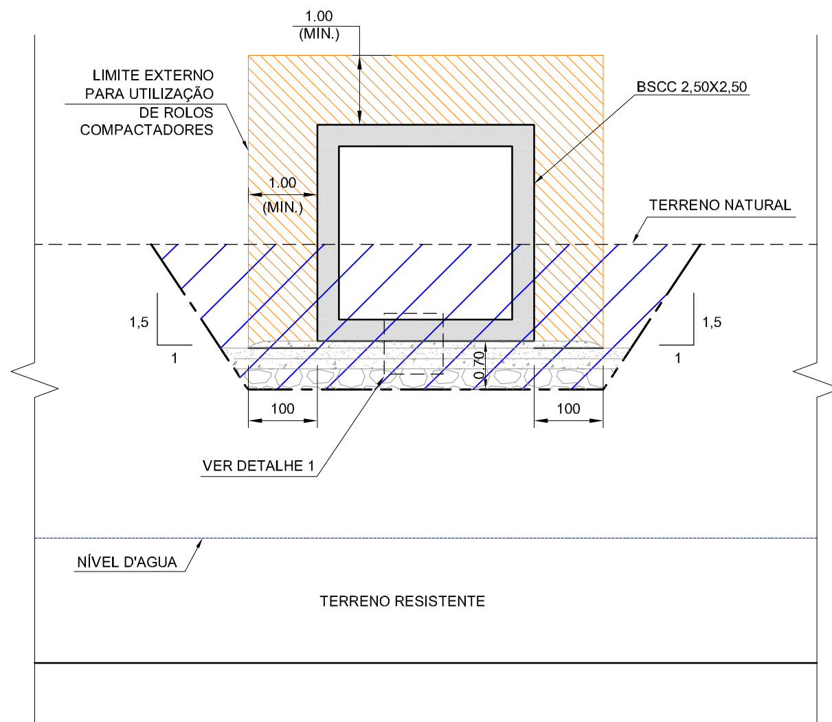
SEÇÃO TÍPICA esc. 1:75
