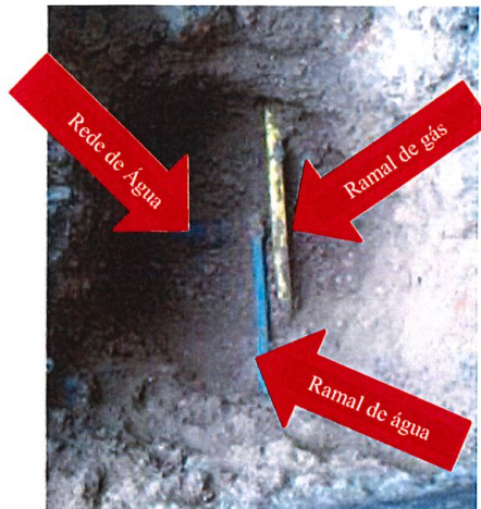
Figura 3 – Ilustra proximidade entre o ramal de gás e a rede/ramal de água
