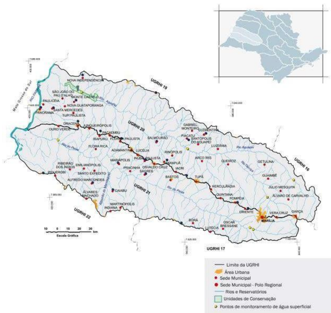
Figura 24 – Bacia Hidrográfica Rio Aguapeí e Rio do Peixe.
